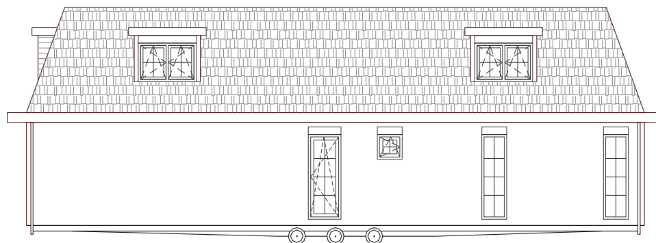
Rechterzij aanzicht
